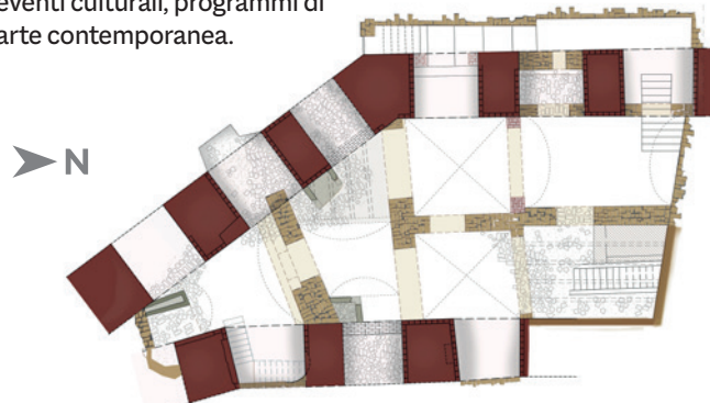
pianta del piano interrato con i resti dell'Acquedotto, a cura di P. Pirozzi
